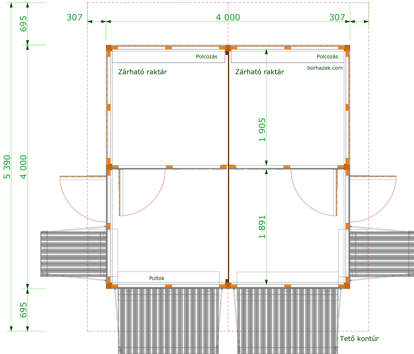
4x4 méteres borház alaprajza I. var.
