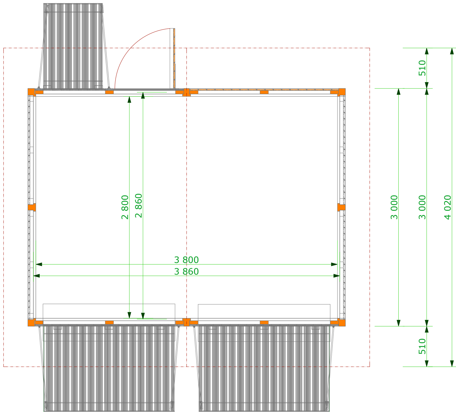
4x3 méteres faház alaprajza
