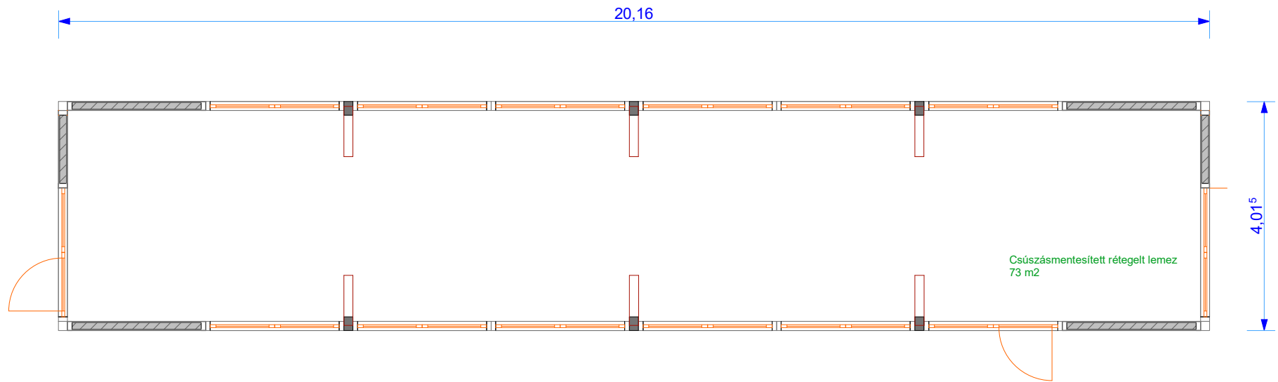
PEZOWOOD 4x20 méteres üvegépület
