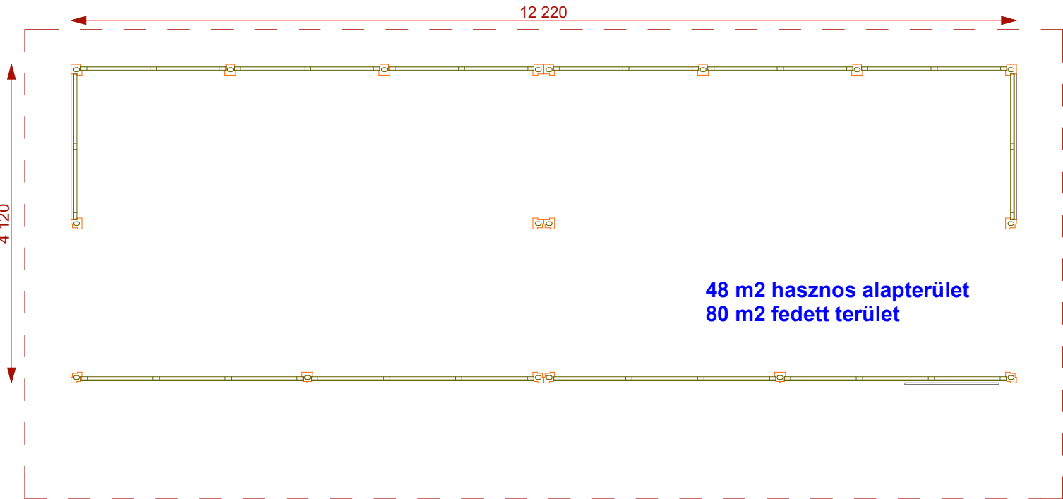
Tető kontúrja
