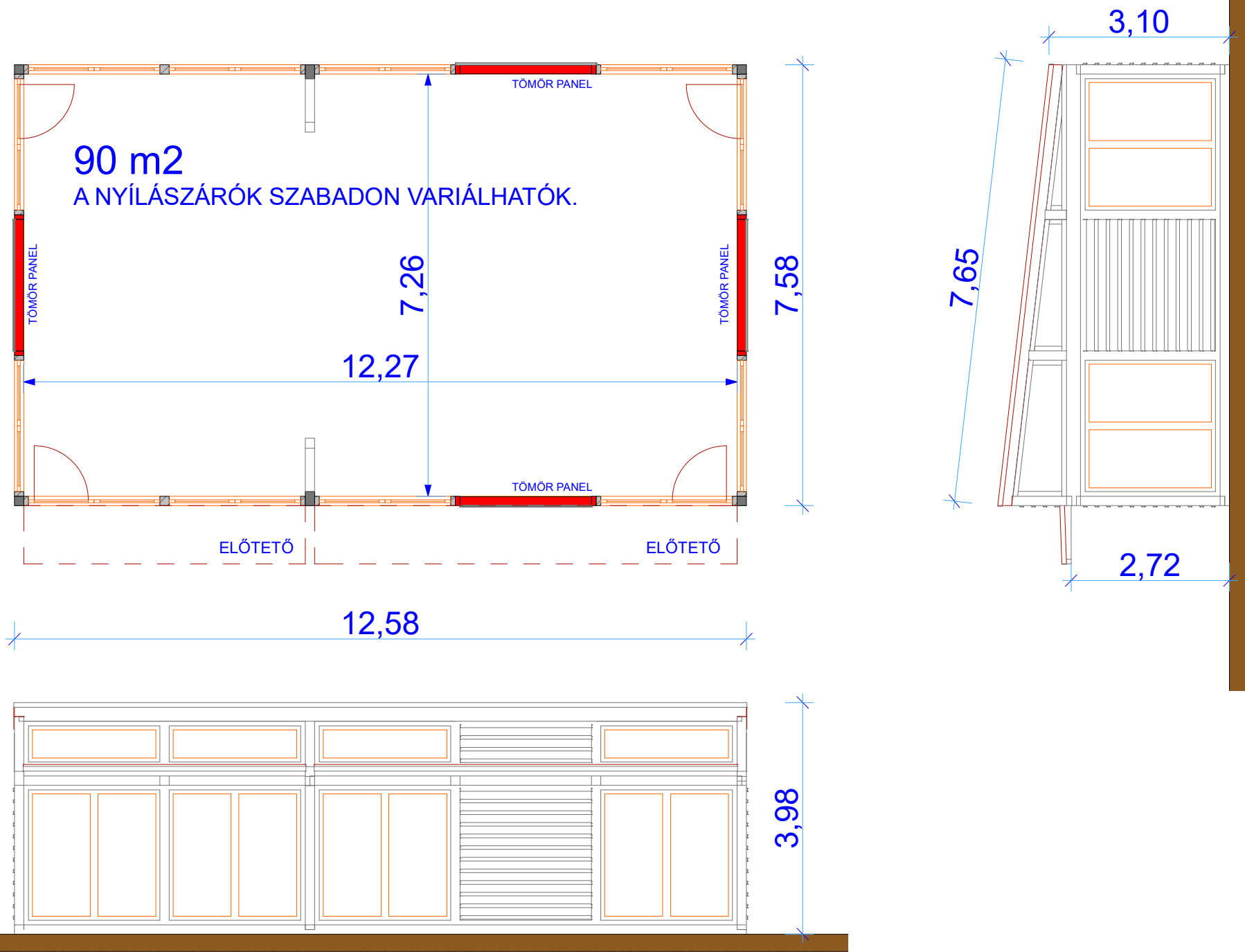
PEZOWOOD NAGY RENDEZVÉNYFAHÁZ ALAPRAJZ, NÉZETI RAJZOK
