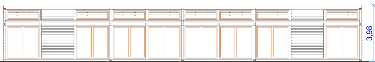
PEZOWOOD NAGY RENDEZVÉNYFAHÁZ ALAPRAJZ, NÉZETI RAJZOK
